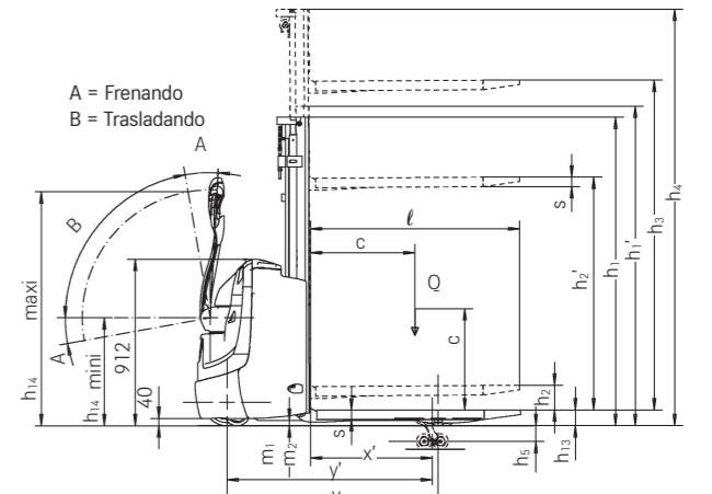
Vista lateral
