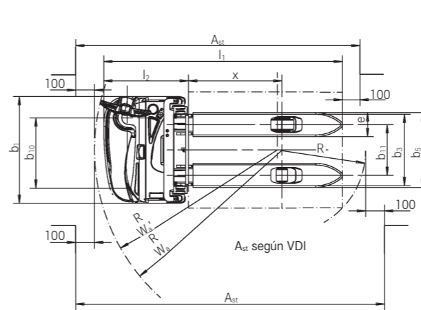
Vista superior
