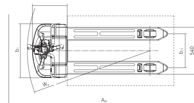
Pôdorys ECH 15
